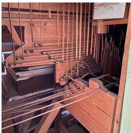
Wellenbrett
