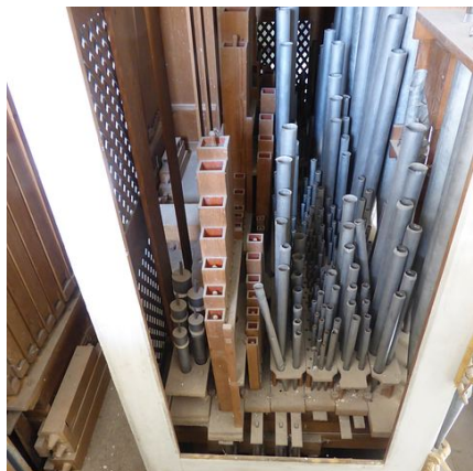
seitlicher Einblick in die Orgel: schwach sichtbar ichtbar die Aufdoppelung der Stöcke im Pedal links und im Manual rechts
