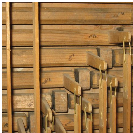
Detail Traktur
