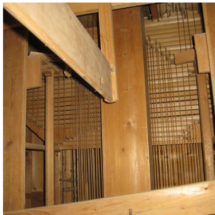
Traktur 2014
